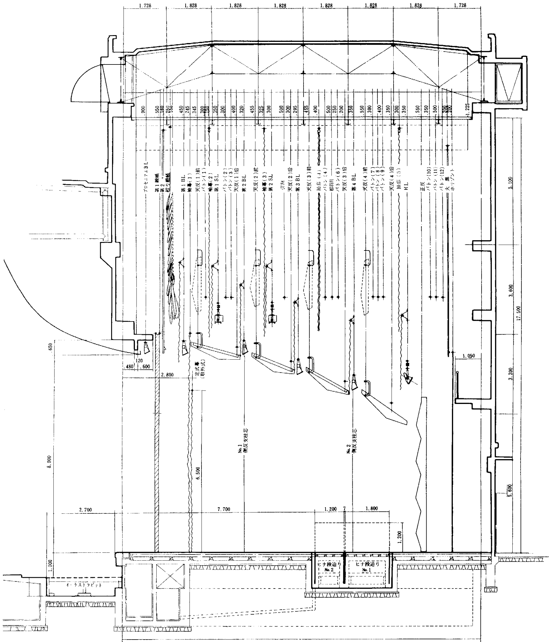
大ホールステージ断面詳細図
